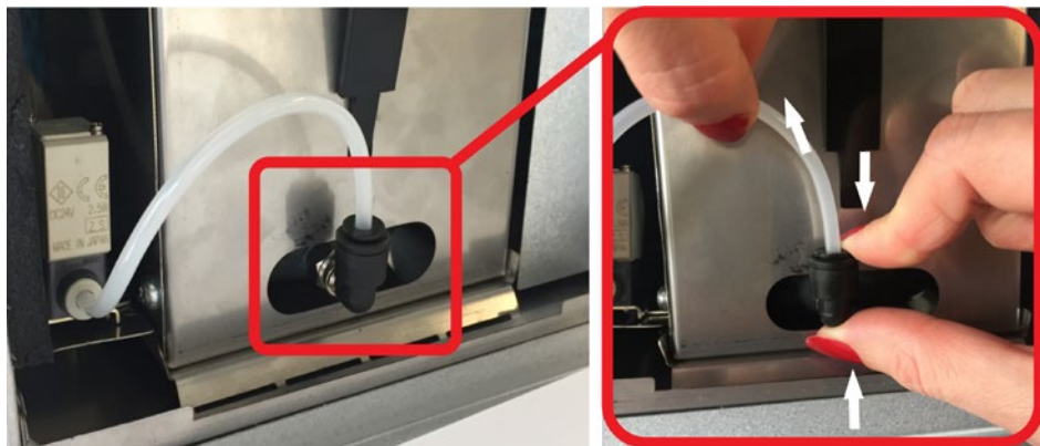
7 pav. Vandens vamzdelio atjungimo schema
