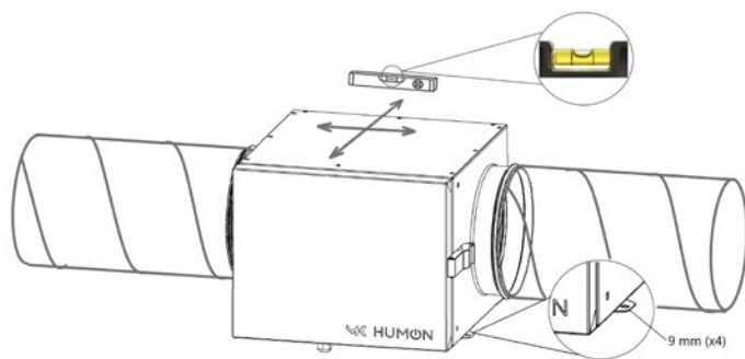
3 pav. Sumontuotas ir išlygintas drėkintuvas HUMON
