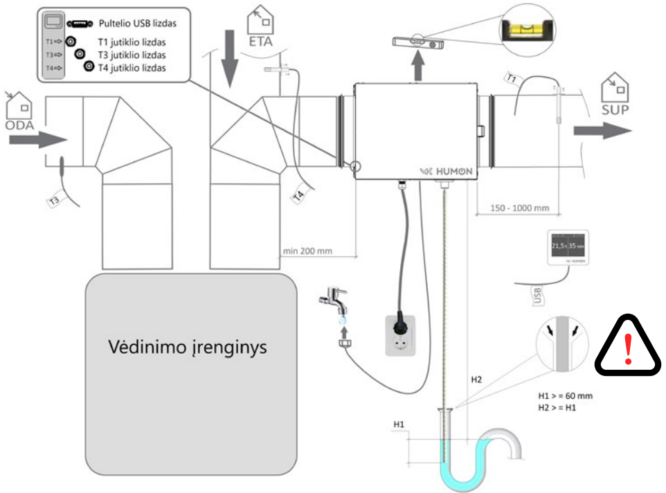
4 pav. HUMON drėkintuvo montavimo schema
